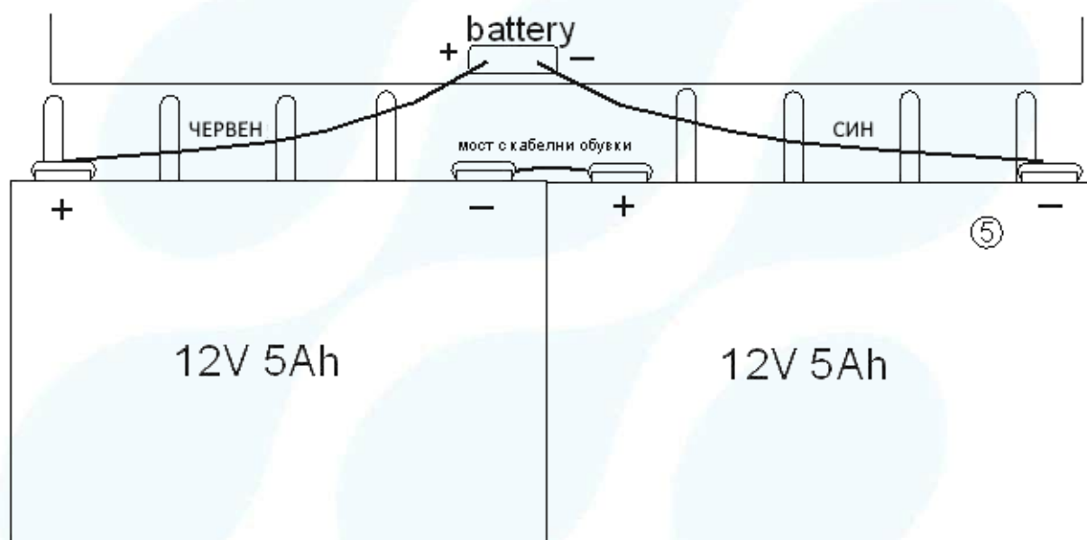
Фиг. 8 - Свързване на акумулаторните батерии
