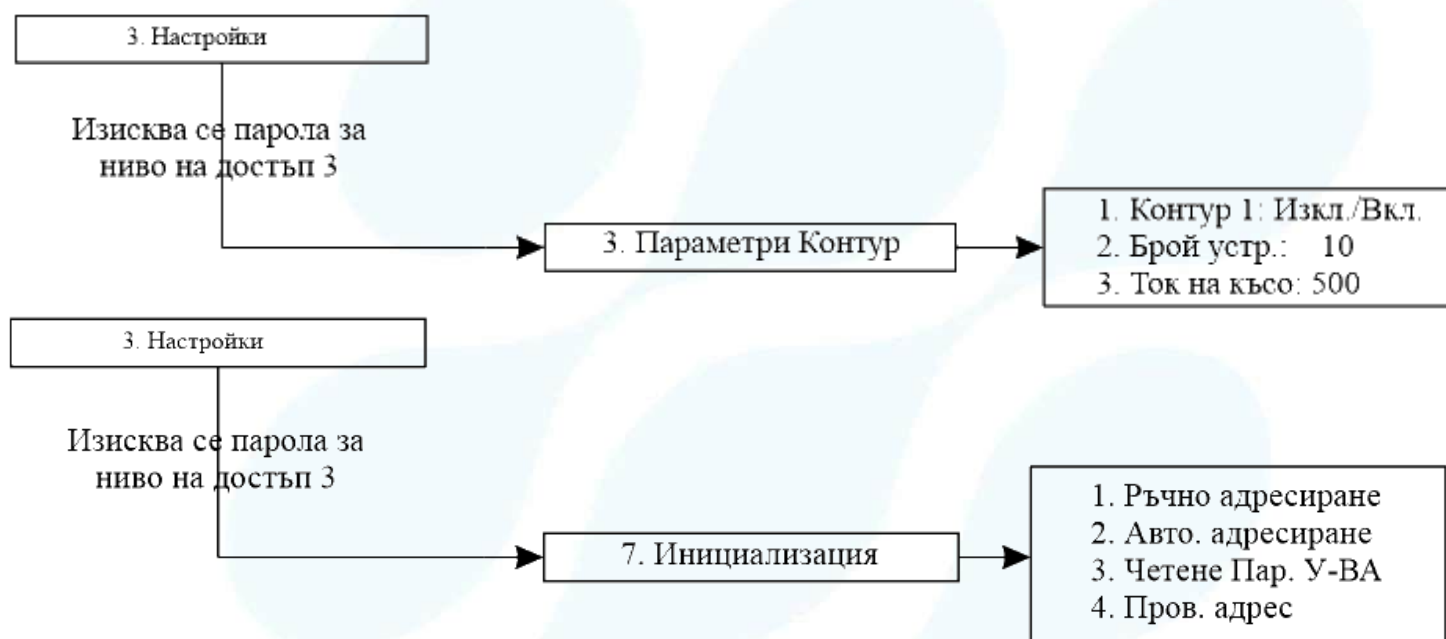
Фиг. 13 – Менюта за промяна параметрите на контураи прочитане на параметрите устройствата
